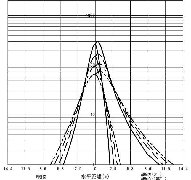
○直射水平面照度 (全光束: 2650 × 1 = 2650lm/台) 照度 (lx) — H1.50m --- H2.00m - - - H2.50m - · - · H3.00m (保守率: 1.00)
