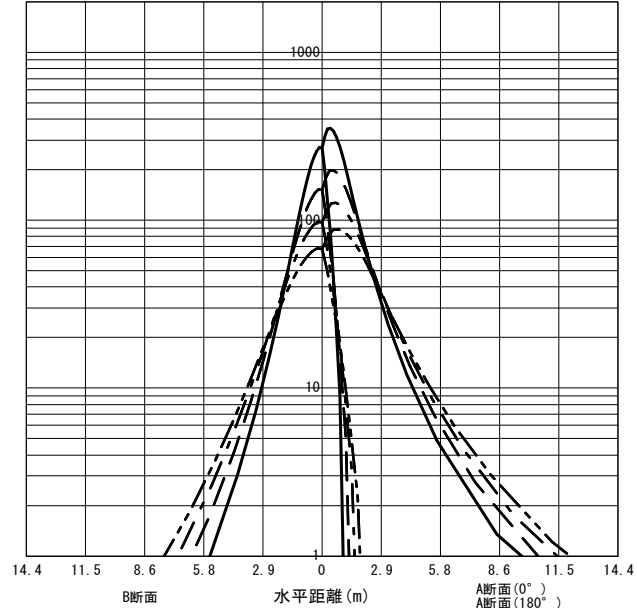
○直射水平面照度 (全光束: 2490 × 1 = 2490lm/台) 照度 (lx) — H1.50m --- H2.00m - - - H2.50m - · - · H3.00m (保守率: 1.00)
