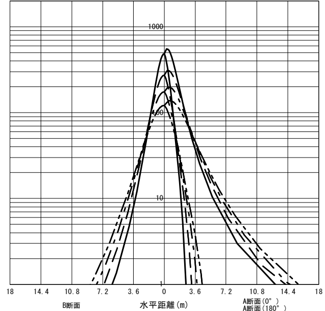
○直射水平面照度 (全光束: 4840 × 1 = 4840lm/台) 照度 (lx) — H1.50m --- H2.00m - - - H2.50m - · - · H3.00m (保守率: 1.00)
