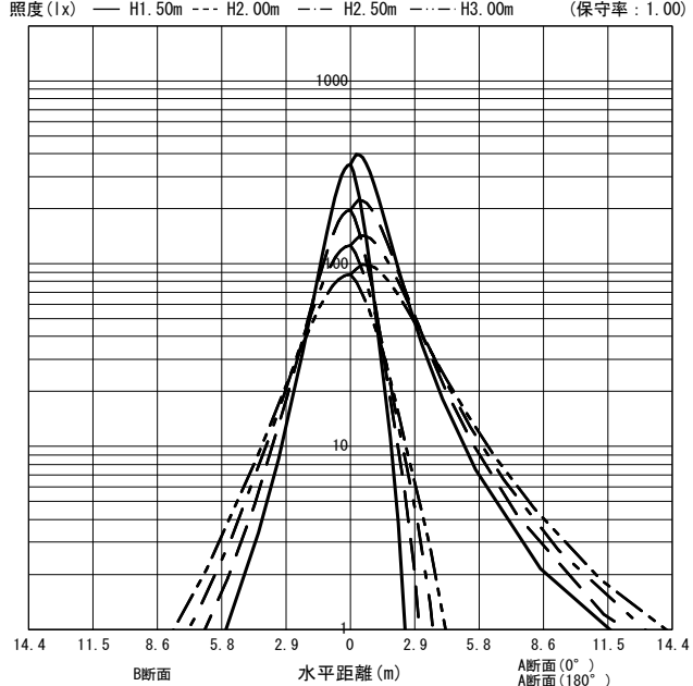
○直射水平面照度 (全光束 : 3480 × 1 = 3480lm/台)
