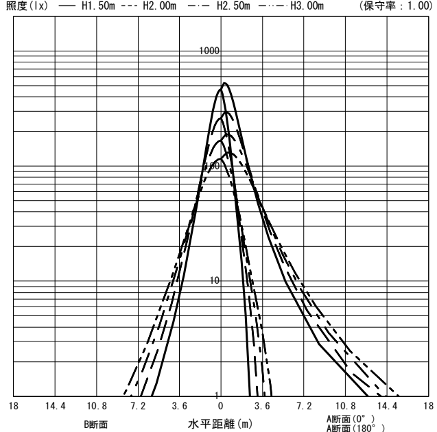
○直射水平面照度 (全光束: 4610 × 1 = 4610lm/台)
