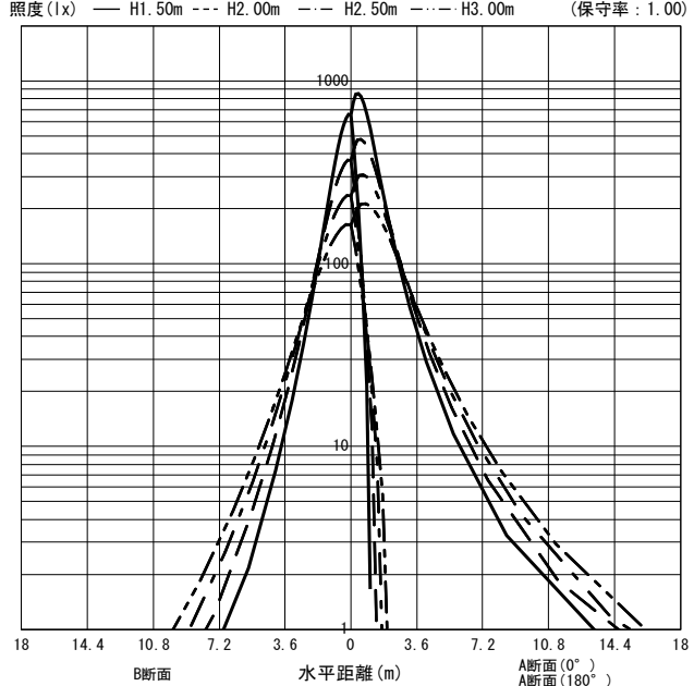
○直射水平面照度 (全光束: 6020 × 1 = 6020lm/台)
