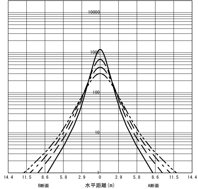
○直射水平面照度 (全光束: 8660 × 1 = 8660lm/台) 照度 (lx) — H1.50m --- H2.00m - - - H2.50m - · - · H3.00m (保守率: 1.00)
