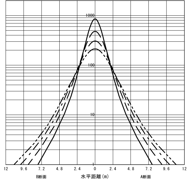
○直射水平面照度 (全光束: 6130 × 1 = 6130lm/台) 照度 (lx) — H1.50m --- H2.00m - - - H2.50m - · - · H3.00m (保守率: 1.00)
