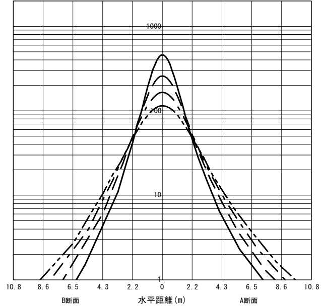
○直射水平面照度 (全光束: 3200 × 1 = 3200lm/台) 照度 (lx) — H1.50m --- H2.00m - - - H2.50m - · - · H3.00m (保守率: 1.00)
