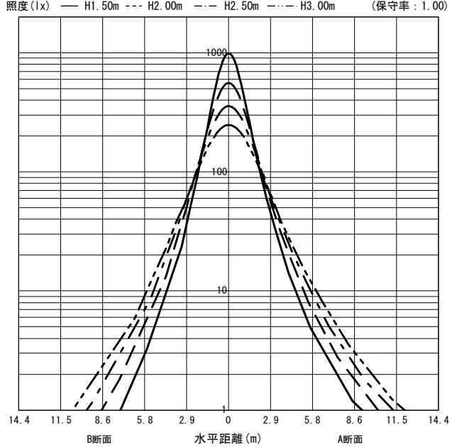
○直射水平面照度 (全光束: 6900 × 1 = 6900lm/台)
