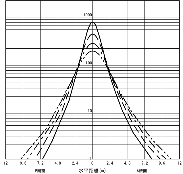
○直射水平面照度 (全光束: 4960 × 1 = 4960lm/台) 照度 (lx) — H1.50m --- H2.00m - - - H2.50m - · - · H3.00m (保守率: 1.00)
