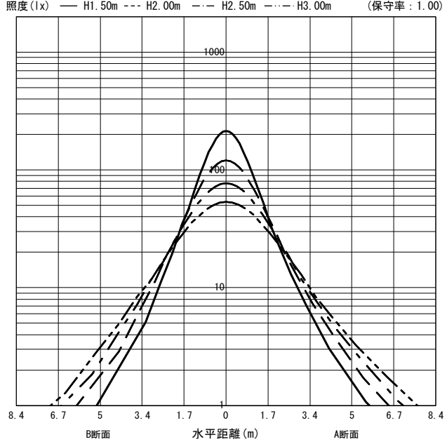
○直射水平面照度 (全光束: 1490 × 1 = 1490lm/台)
