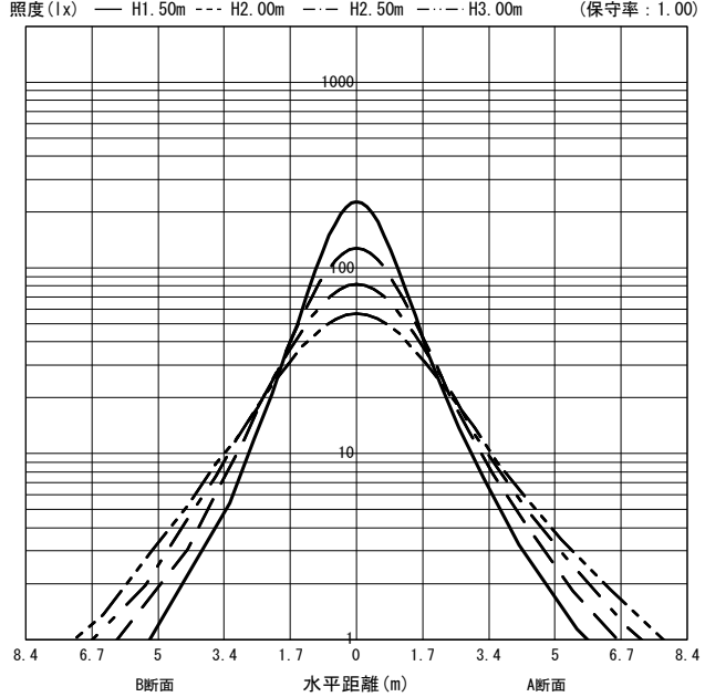
○直射水平面照度 (全光束: 1580 × 1 = 1580lm/台)
