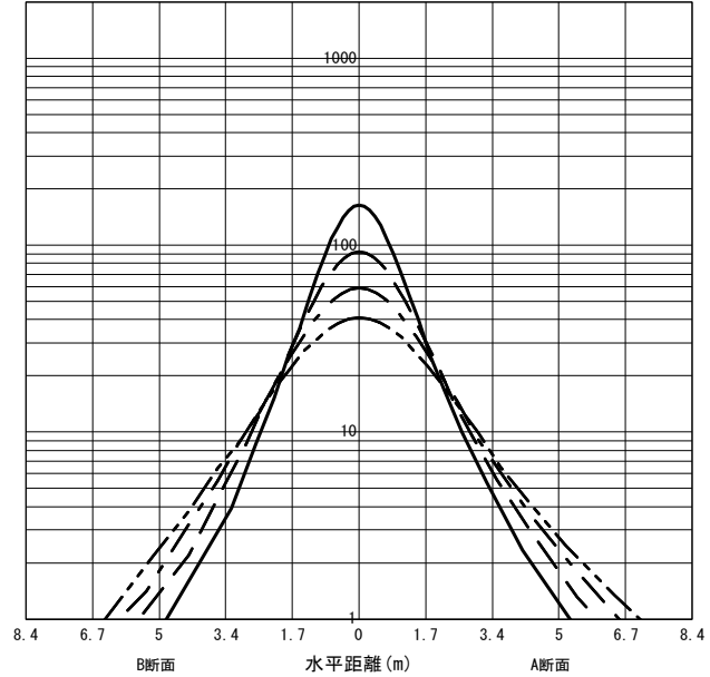
○直射水平面照度 (全光束: 1140 × 1 = 1140lm/台) 照度 (lx) — H1.50m --- H2.00m - - - H2.50m - · - · H3.00m (保守率: 1.00)
