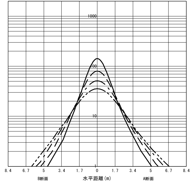
○直射水平面照度 (全光束: 990 × 1 = 990lm/台) 照度 (lx) — H1.50m --- H2.00m - - - H2.50m - · - - H3.00m (保守率: 1.00)
