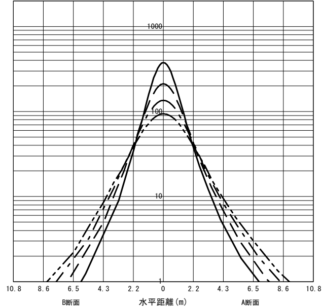
○直射水平面照度 (全光束: 2620 × 1 = 2620lm/台) 照度 (lx) — H1.50m --- H2.00m - - - H2.50m - · - · H3.00m (保守率: 1.00)
