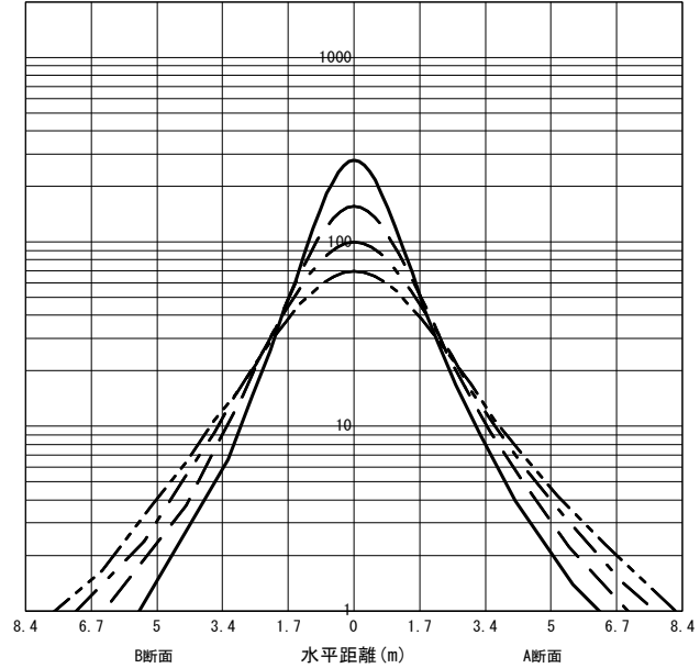
○直射水平面照度 (全光束: 1930 × 1 = 1930lm/台) 照度 (lx) — H1.50m --- H2.00m - - - H2.50m - · - · H3.00m (保守率: 1.00)
