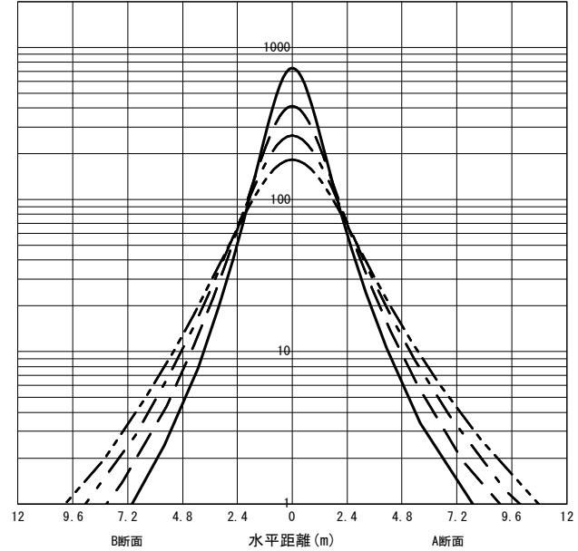
○直射水平面照度 (全光束: 4990 × 1 = 4990lm/台) 照度 (lx) — H1.50m --- H2.00m - - - H2.50m - · - · H3.00m (保守率: 1.00)
