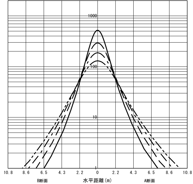
○直射水平面照度 (全光束: 3550 × 1 = 3550lm/台) 照度 (lx) — H1.50m --- H2.00m - - - H2.50m - · - · H3.00m (保守率: 1.00)
