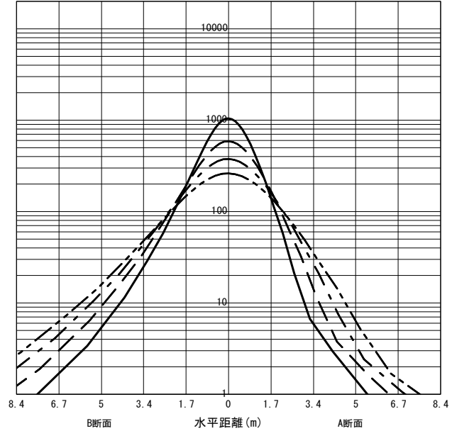
○直射水平面照度 (全光束: 6070 × 1 = 6070lm/台) 照度 (lx) — H1.50m --- H2.00m - - - H2.50m - · - · H3.00m (保守率: 1.00)
