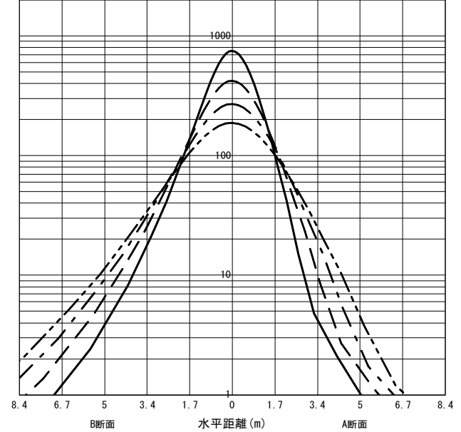
○直射水平面照度 (全光束: 4360 × 1 = 4360lm/台) 照度 (lx) —— H1.50m --- H2.00m - - - H2.50m - · - · H3.00m (保守率: 1.00)
