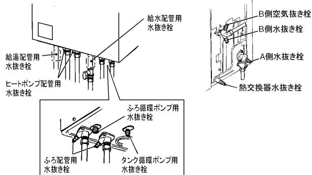
〈貯湯タンクユニット〉
