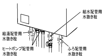
〈貯湯タンクユニット〉
