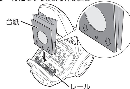
レール
