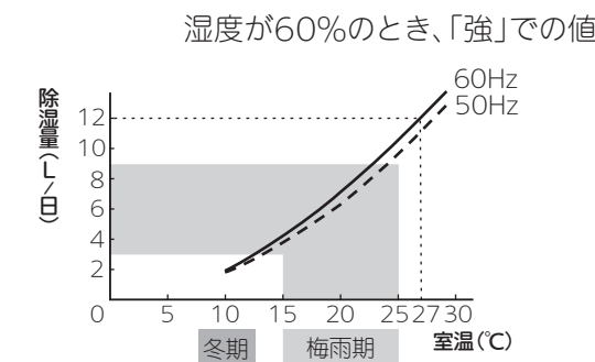
グラフの除湿量は、一定の室温・湿度にて測定した値であり、実際の使用条件とは異なります。
