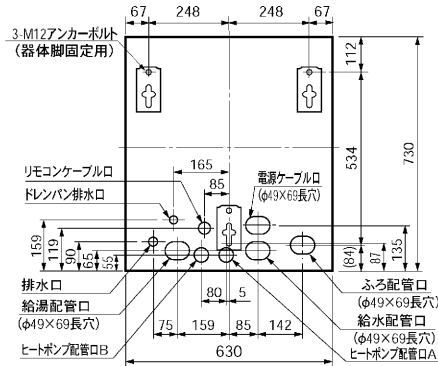
配管、アンカーボルト位置上面透視図 (370L、460L)
