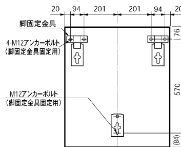
脚固定使用時アンカーボルト位置 上面透視図 (370L、460L)
