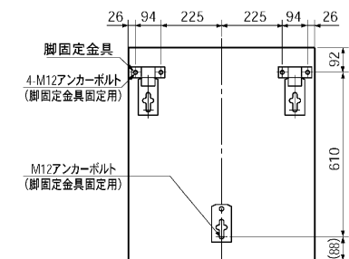
脚固定使用時アンカーボルト位置 上面透視図 (460Lローボディ)
