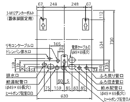
配管、アンカーボルト位置上面透視図 (370L、460L)
