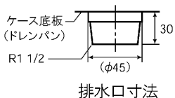
排水口寸法
