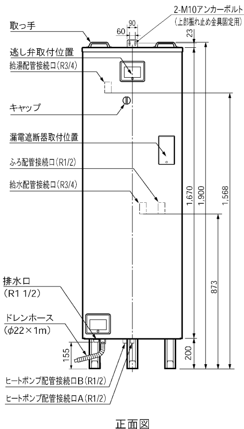
正面図
