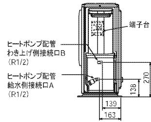
配管位置 右側図
