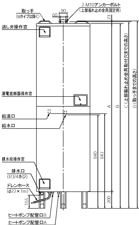
正面図
