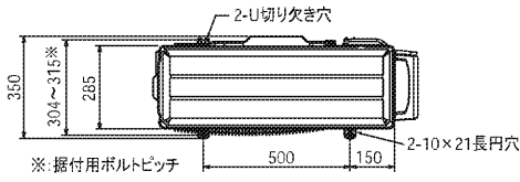
上面図
