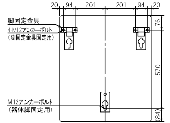
脚固定金具使用時 アンカーボルト位置上面透視図 (370L/460L)
