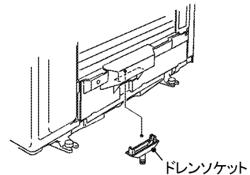
ドレンソケットの取り付け
