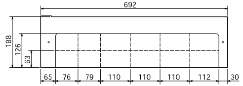
側面カバー(左)
