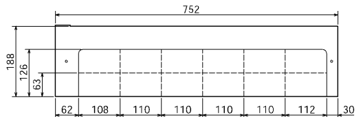
側面カバー(左)
