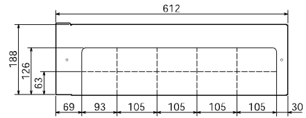
側面カバー(右)
