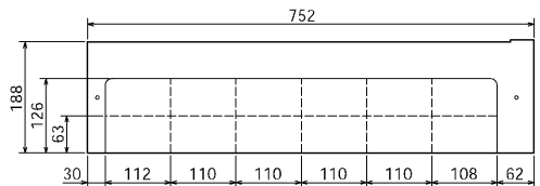
側面カバー(左)
