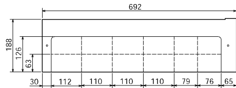
側面カバー(左)
