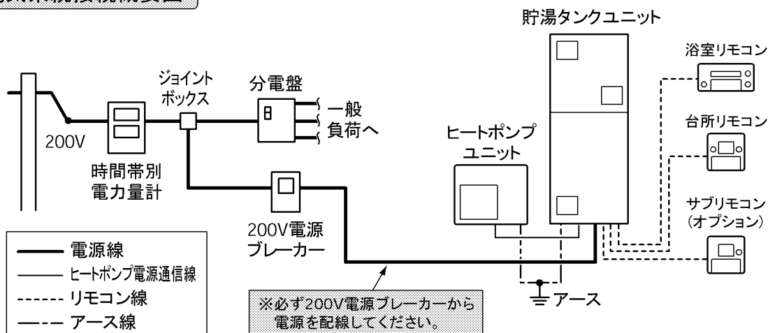
電気系統接続概要図
