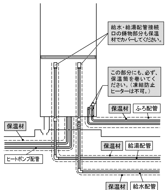
貯湯タンクユニット
