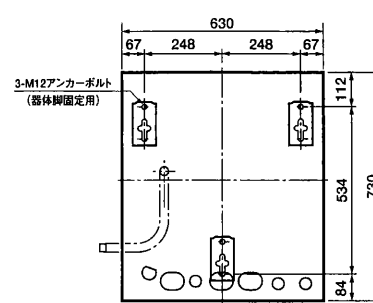
アンカーボルト位置:上面透視図
