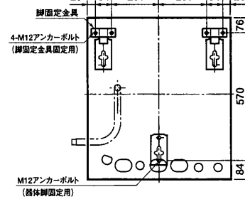
脚固定金具使用時:上面透視図
