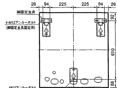
脚固定金具使用時：上面透視図 〔550L、ローボディ用〕
