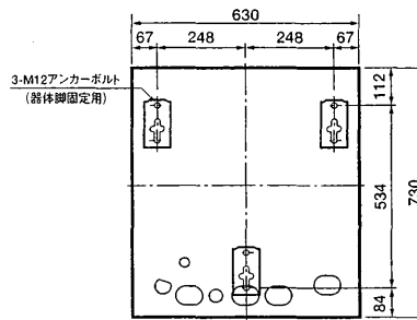
アンカーボルト位置：上面透視図 〔370L、460L用〕
