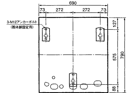
アンカーボルト位置：上面透視図 〔550L、ローボディ用〕
