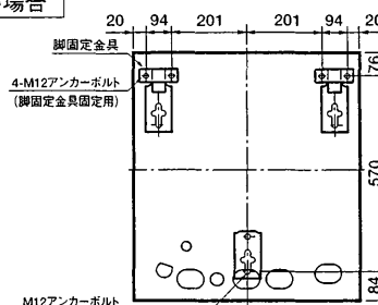
脚固定金具使用時：上面透視図 〔370L、460L用〕
