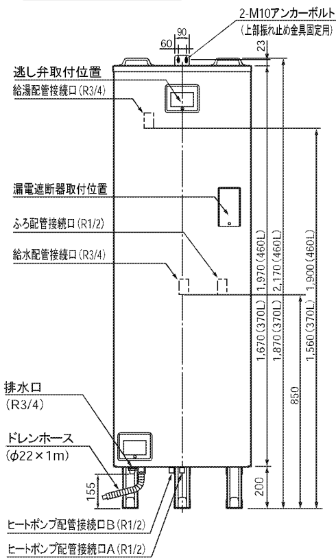
正面図
