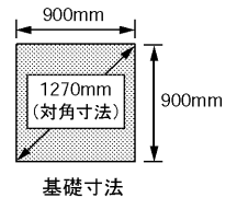
基礎寸法
