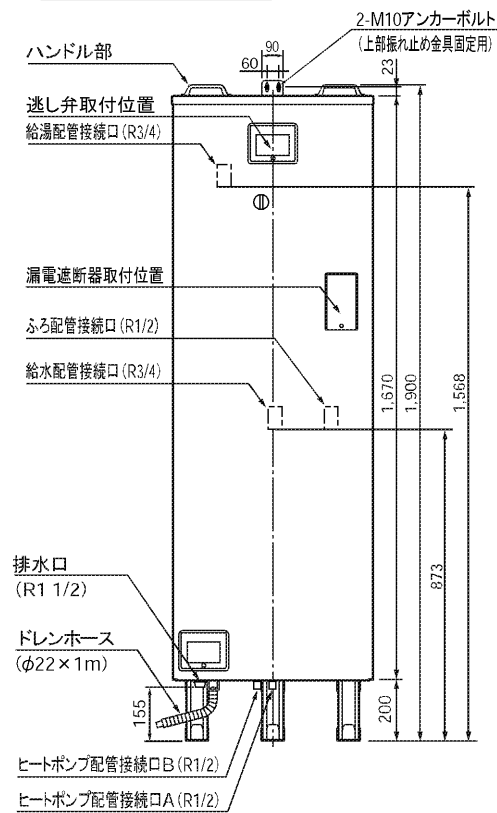
正面図
