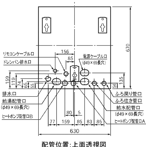
配管位置: 上面透視図
