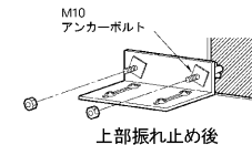
上部振れ止め後
