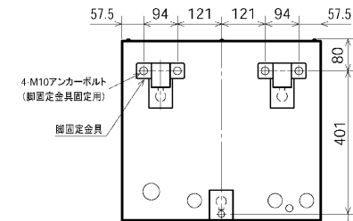
脚固定金具使用時:上面透視図 [200L機種]
