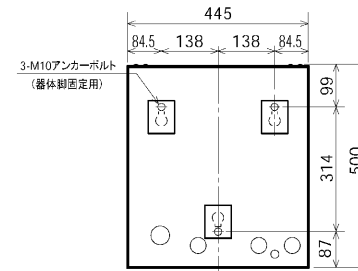
アンカーボルト位置:上面透視図 [150L機種]
