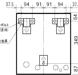
脚固定金具使用時:上面透視図 [150L機種]
