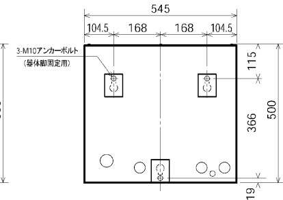
アンカーボルト位置:上面透視図 [200L機種]
