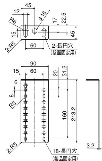
上部振れ止め金具寸法図(単位:mm)
