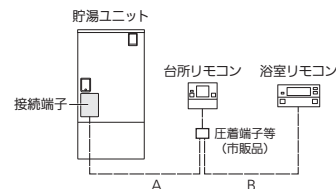
接続例2
