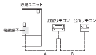
接続例1(渡り配線時 当社推奨接続)
