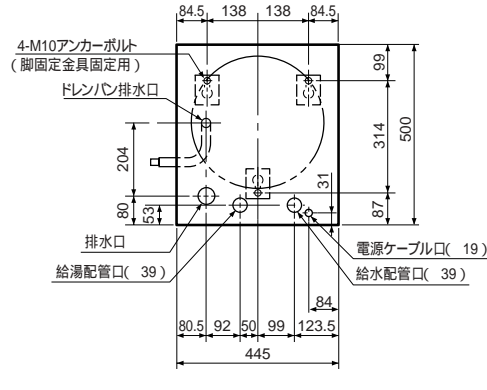
配管、アンカーボルト位置上面透視図 (SRT-1518)
