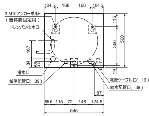
配管、アンカーボルト位置上面透視図 (SRT-2018)
