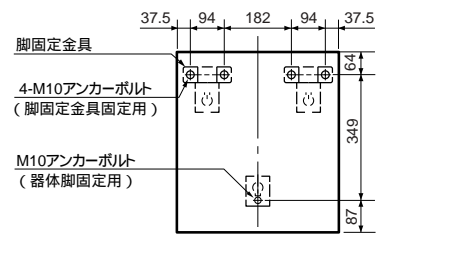
脚固定使用時アンカーボルト位置上面透視図 (SRT-1518)
