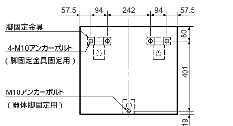
脚固定使用時アンカーボルト位置上面透視図 (SRT-2018)
