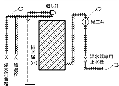
(1)凍結防止ヒーターによる方法
