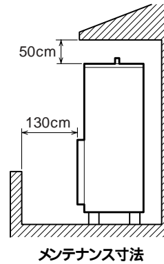
メンテナンス寸法
