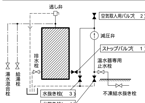
(3)水抜きによる方法
