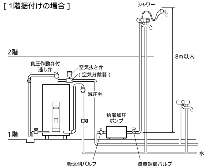
[1階据付けの場合]
