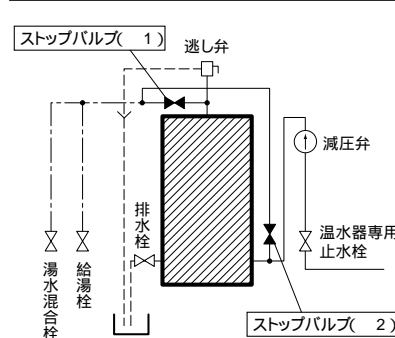
(2)少量の水を流し続ける方法
