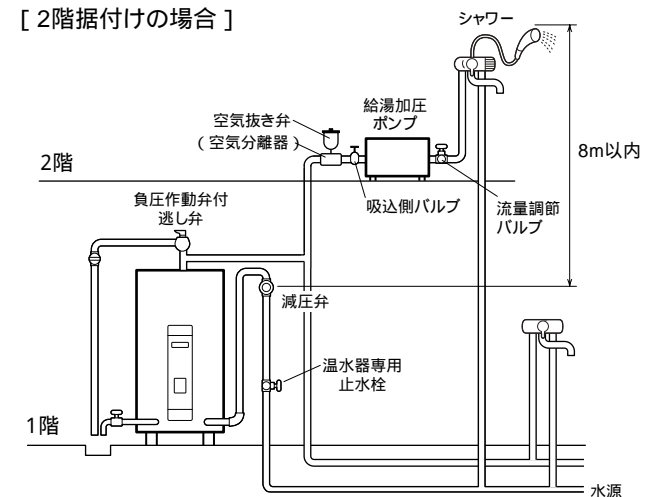
[2階据付けの場合]
