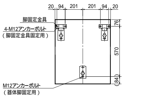
脚固定使用時アンカーボルト位置上面透視図 (SRG-3768, SRG-4668)
