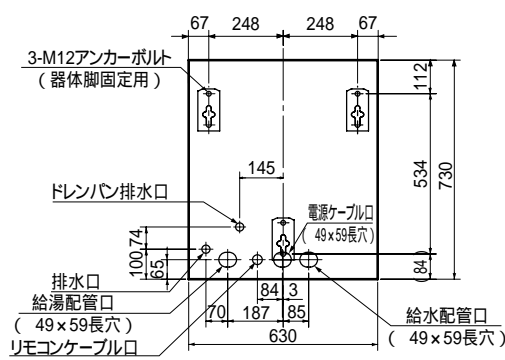
配管、アンカーボルト位置上面透視図 (SRG-3768, SRG-4668)
