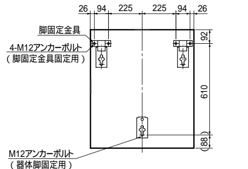
脚固定使用時アンカーボルト位置上面透視図 (SRG-5568)
