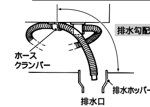
図2 温水器が排水口から近い場合
