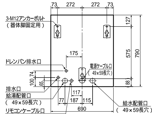
配管、アンカーボルト位置上面透視図 (SRT-5568U)
