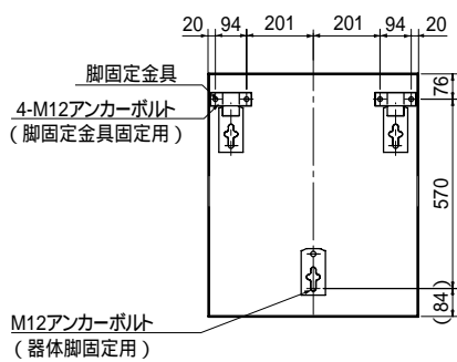
脚固定使用時アンカーボルト位置上面透視図 (SRT-3768U, SRT-4668U)
