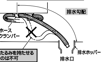
温水器が排水口から遠い場合
