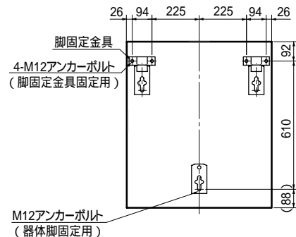
脚固定使用時アンカーボルト位置上面透視図 (SRT-5568U)
