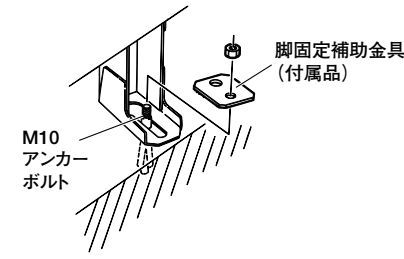
アンカーボルト固定後
