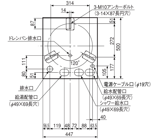
配管、アンカーボルト位置上面透視図 (SRC-151AR)
