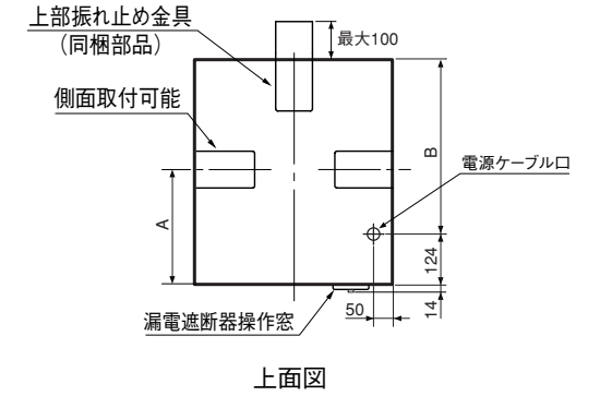
上面図
