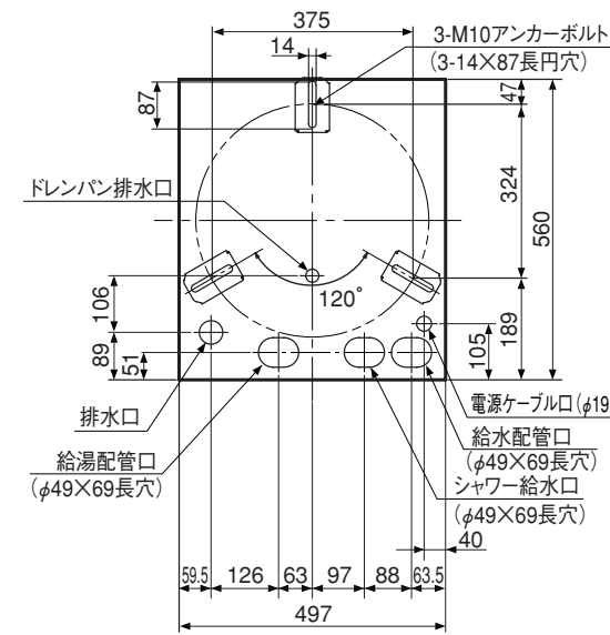
配管、アンカーボルト位置上面透視図 (SRC-201AR)
