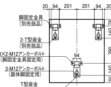
標準施工ができない場合 アンカーボルト位置上面透視図 (SRG-466B)
