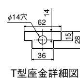
T型座金詳細図
