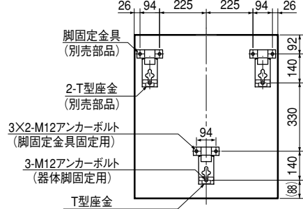
標準施工ができない場合 アンカーボルト位置上面透視図 (SRG-556B)
