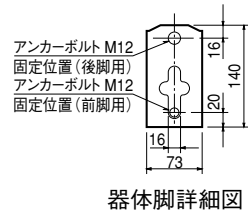
器体脚詳細図
