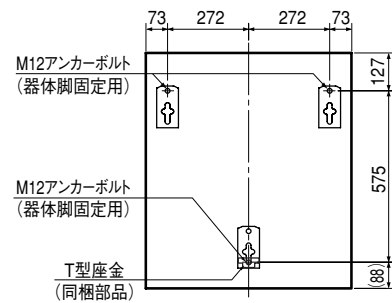
標準施工時 アンカーボルト位置上面透視図 (SRG-556B)
