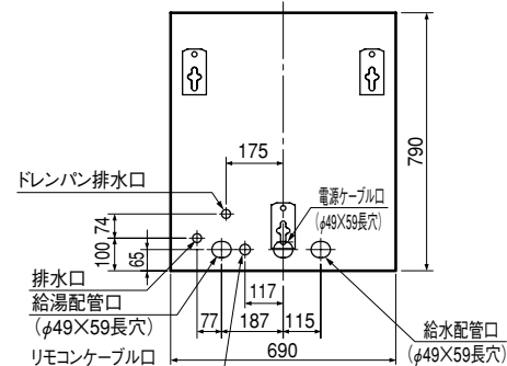
配管位置上面透視図 (SRG-556B)
