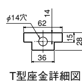
T型座金詳細図
