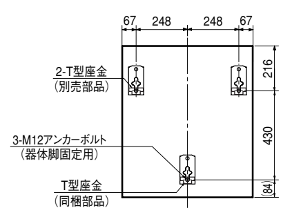
標準施工ができない場合 アンカーボルト位置上面透視図 (SRG-376B)
