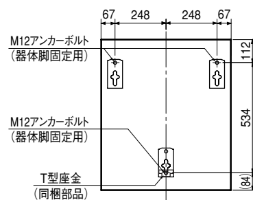
標準施工時 アンカーボルト位置上面透視図 (SRG-376B, SRG-466B)
