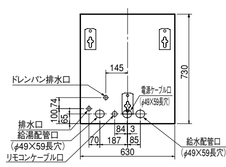
配管位置上面透視図 (SRG-376B, SRG-466B)
