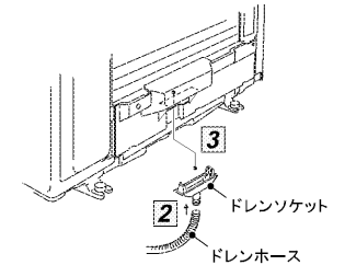
ドレンソケットの取り付け
