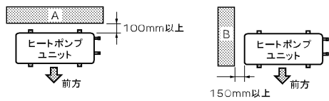
ヒートポンプユニット（上から見た図）
