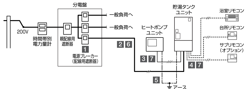
接続図2
