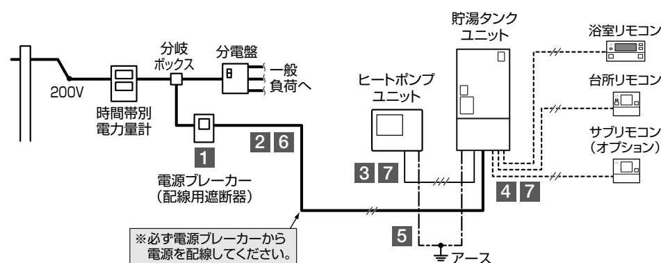
接続図2
