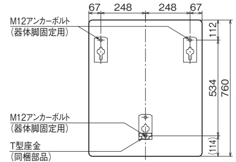
標準施工時 アンカーボルト位置上面透視図
